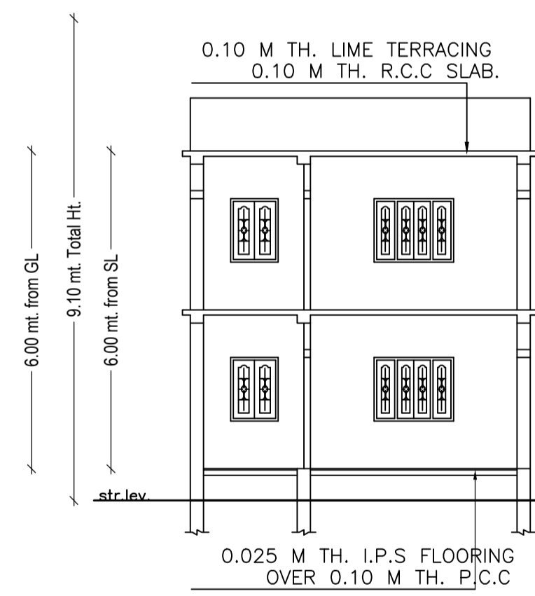
SECTION ON: <1-1> SCALE : (1:100)
