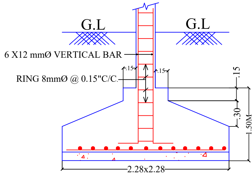
SECTION OF FOOTING - F1
