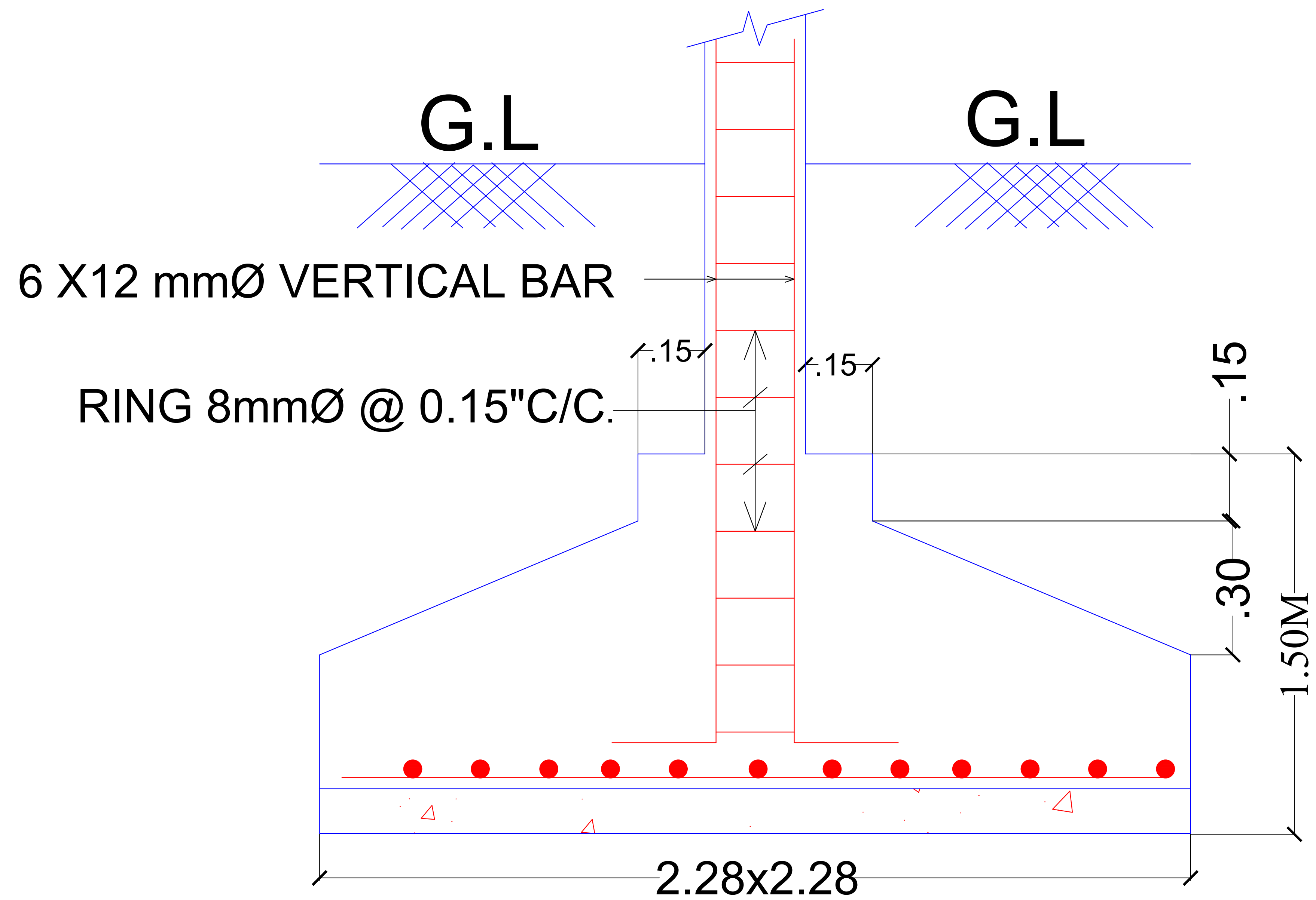
SECTION OF FOOTING - F1
