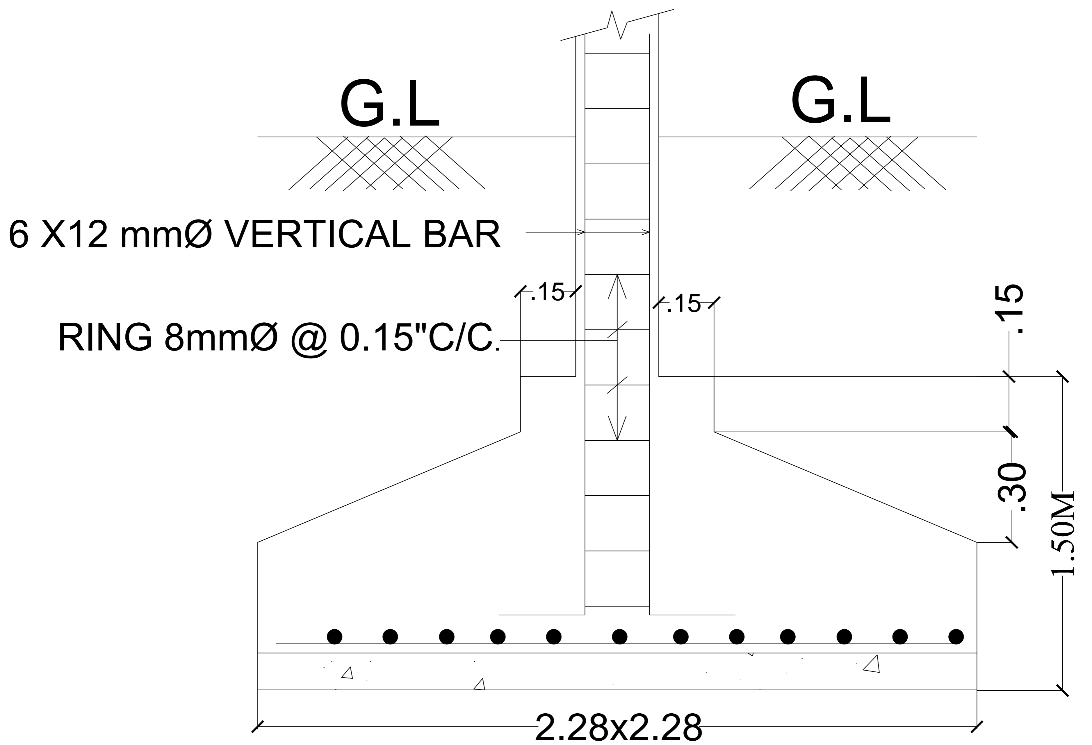
SECTION OF FOOTING - F1
