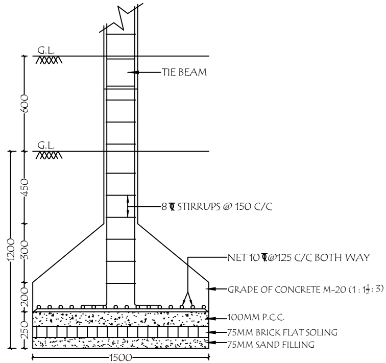
SECTION X X Scale - N.T.S.
