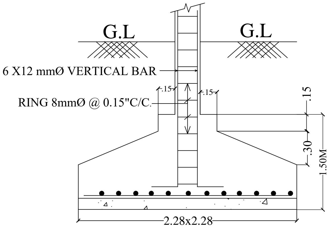
SECTION OF FOOTING - F1
