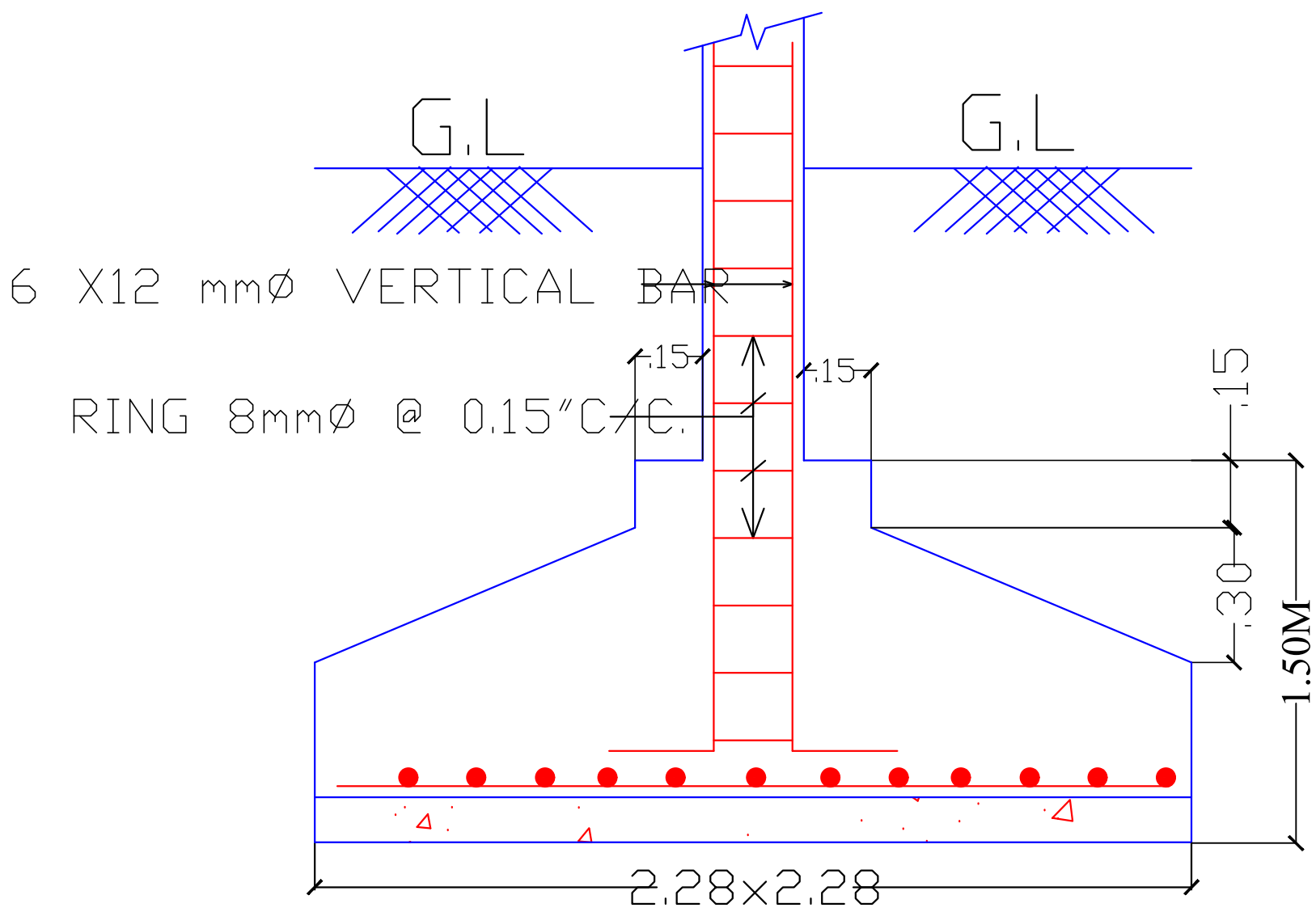
SECTION OF FOOTING - F1
