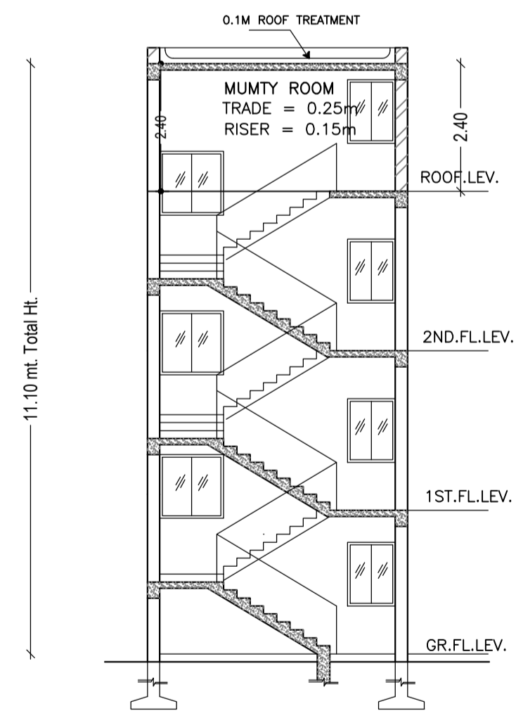
SCALE : 1:100
