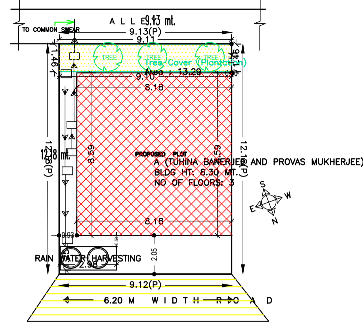
SITE PLAN SCALE:1:100 (Scale - 1:200)
