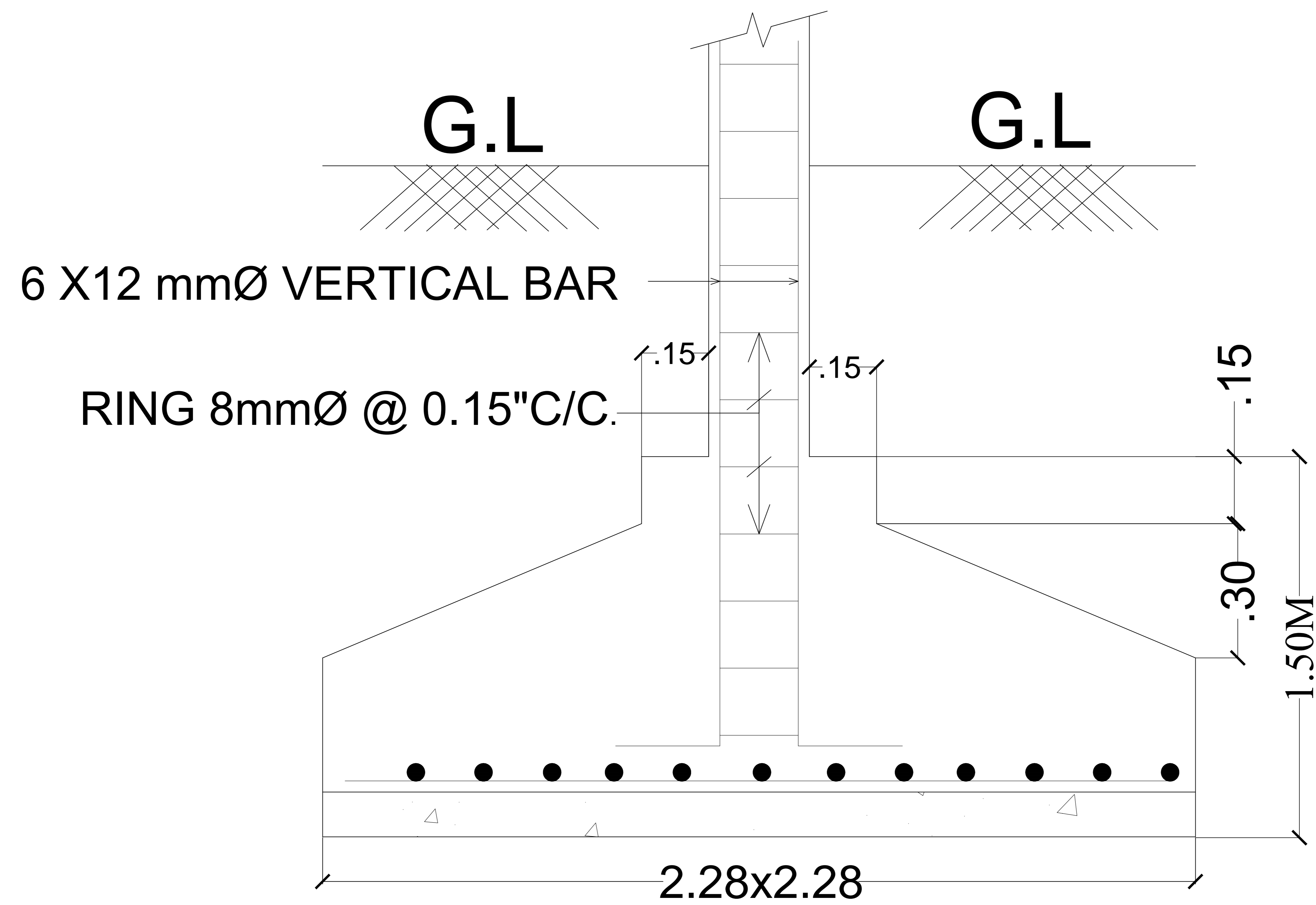
SECTION OF FOOTING - F1
