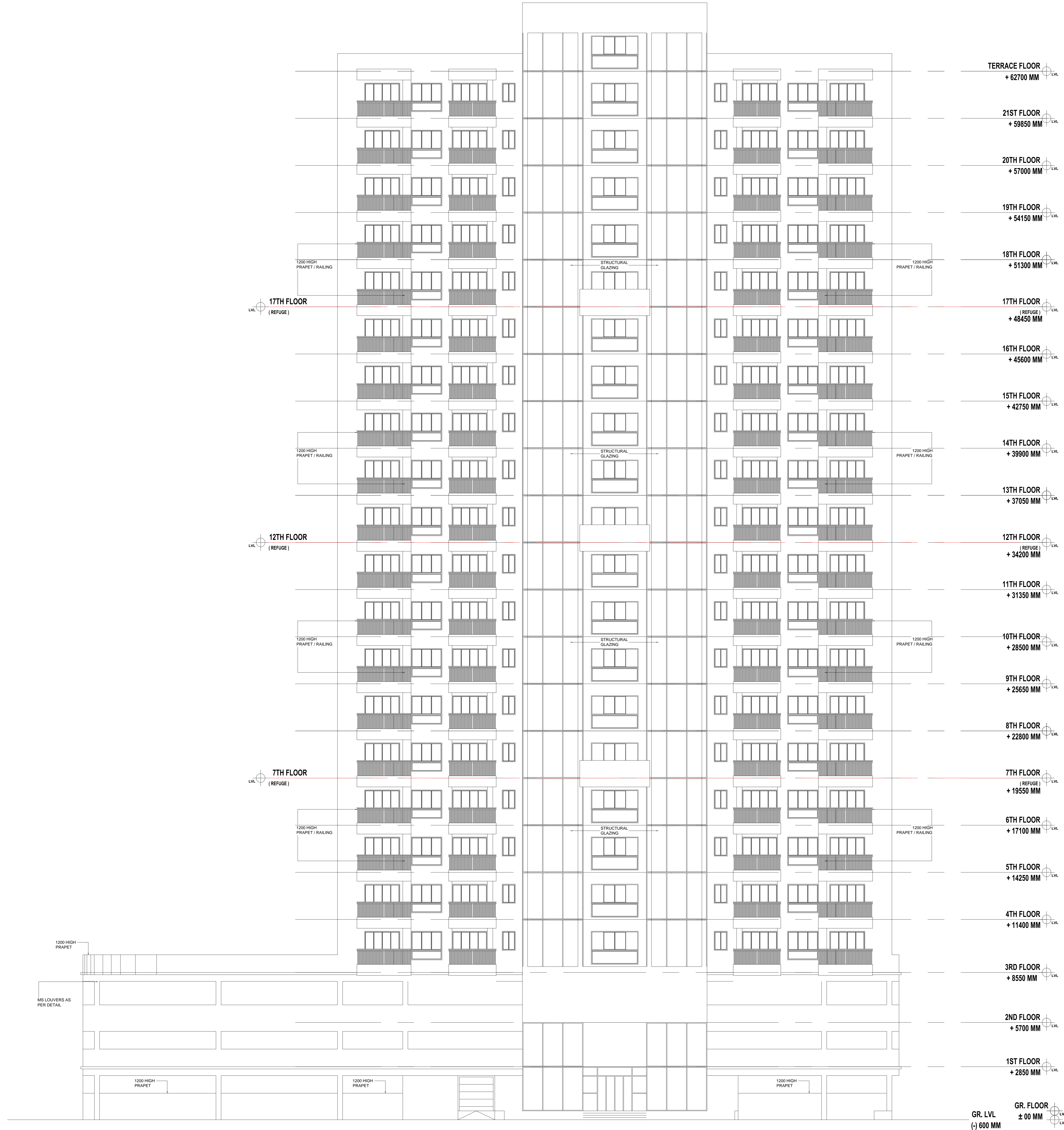
ELEVATION XX'
