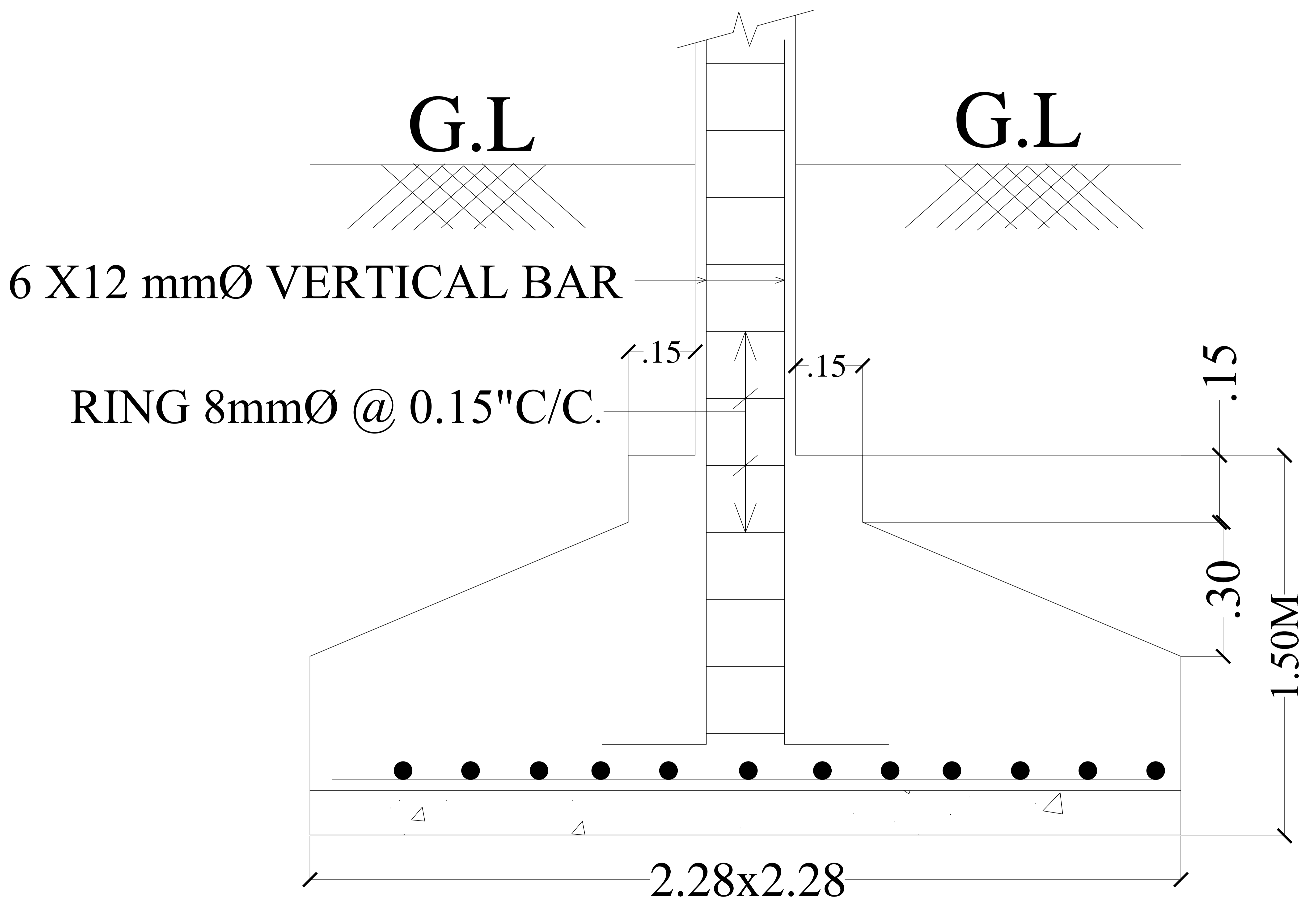
SECTION OF FOOTING - F1
