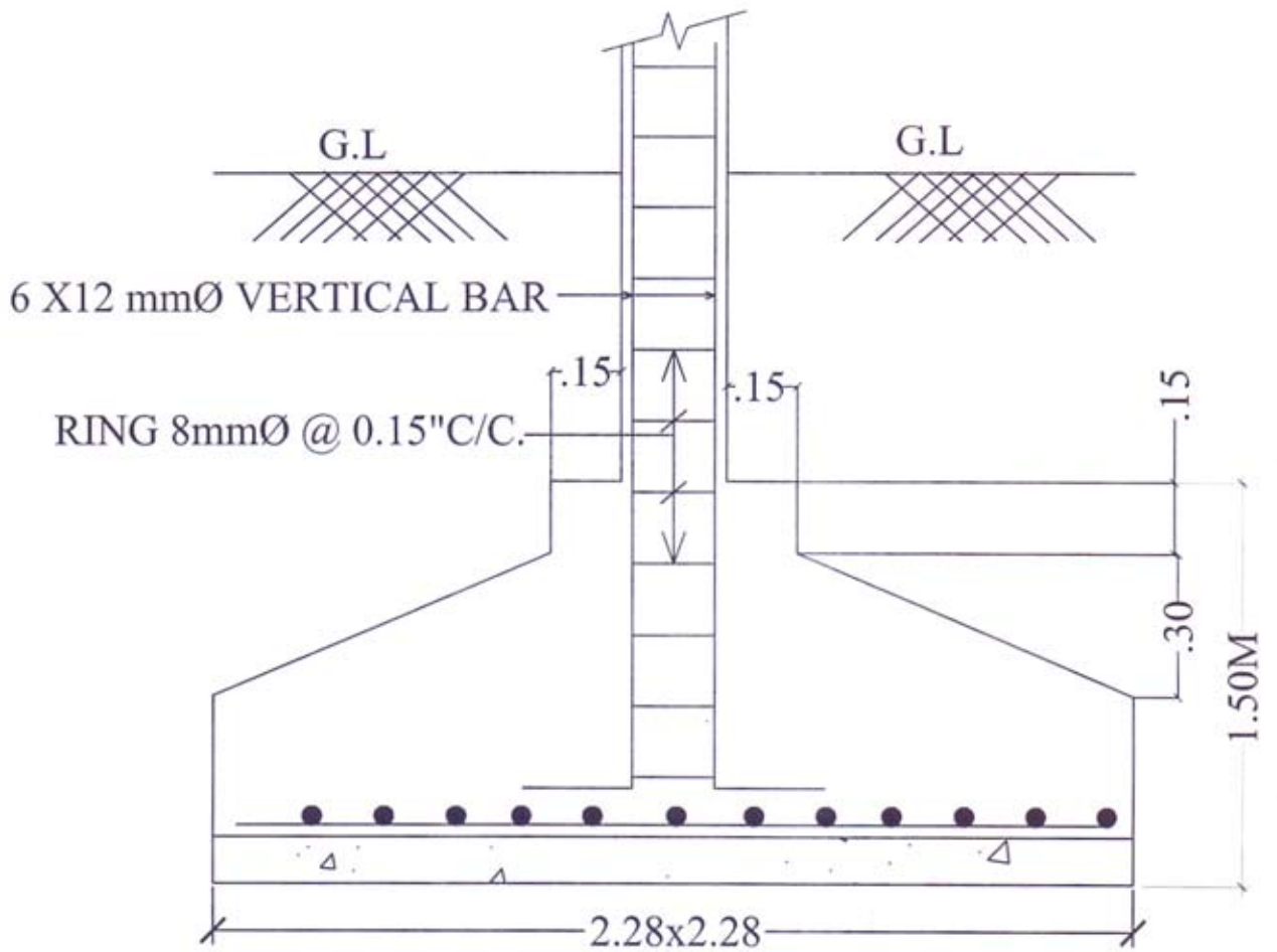
SECTION OF FOOTING - F1
