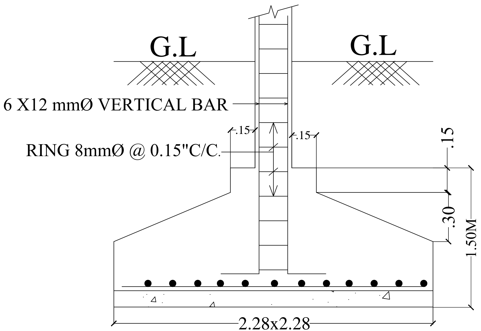
SECTION OF FOOTING - F1
