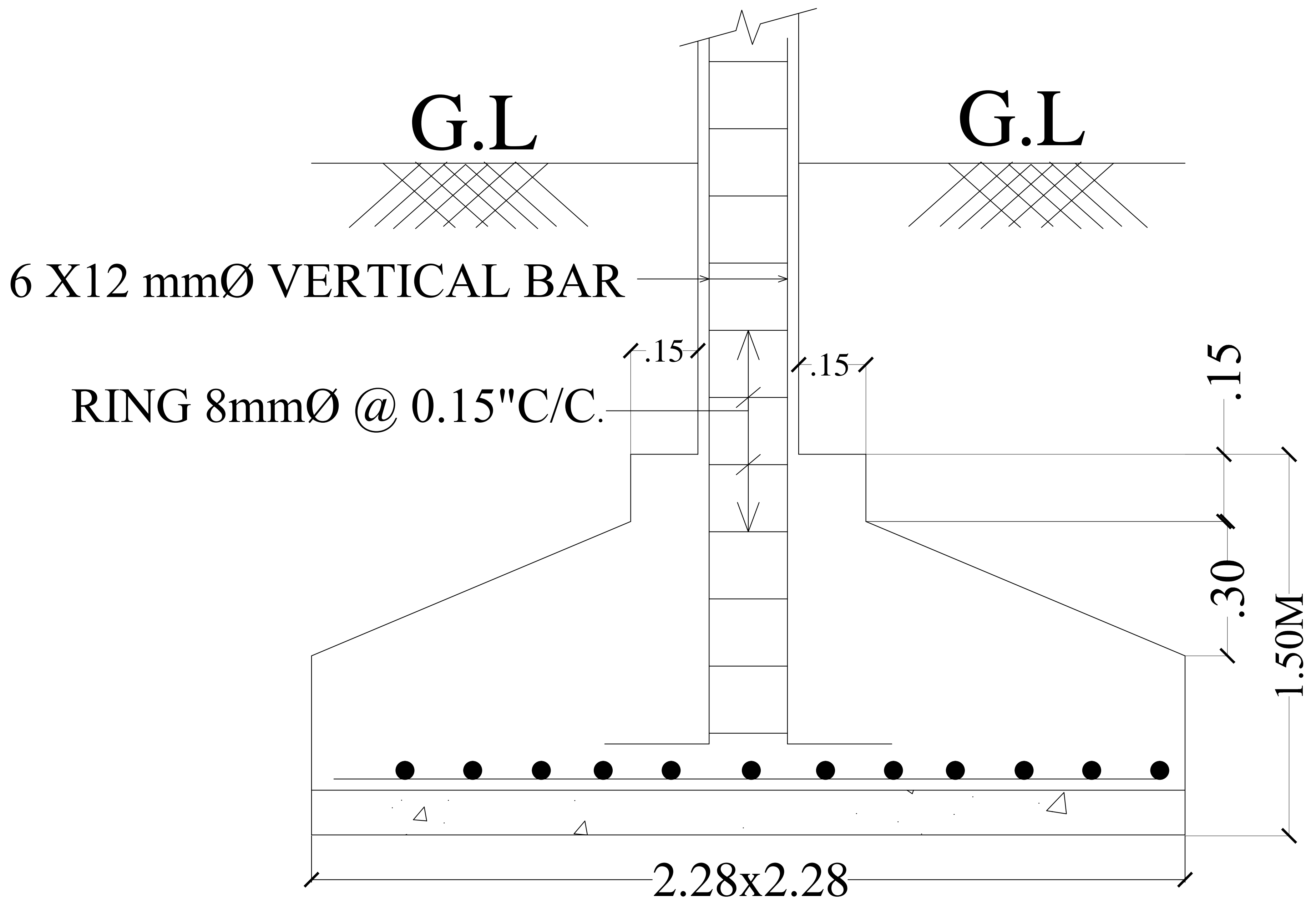
SECTION OF FOOTING - F1
