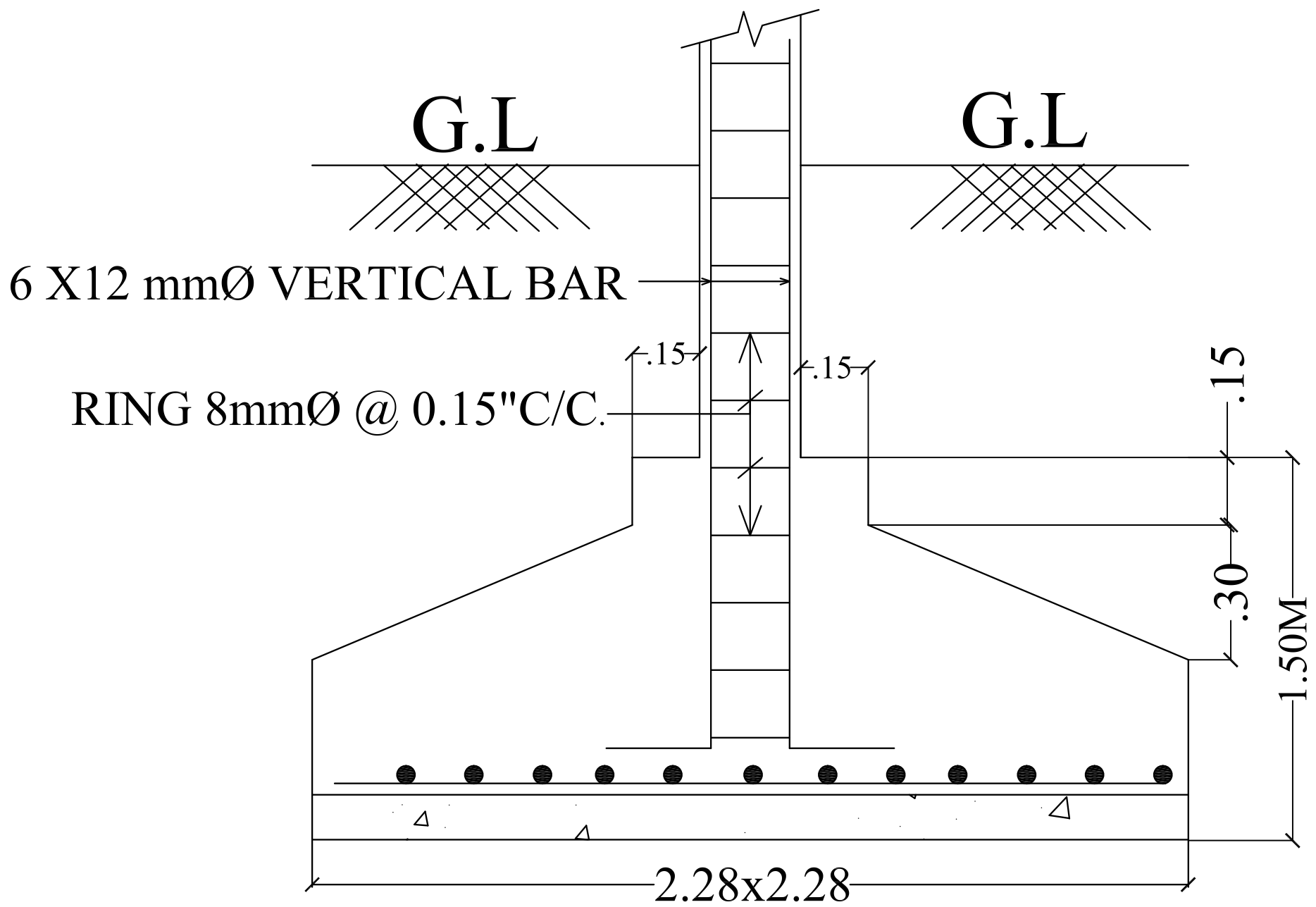
SECTION OF FOOTING - F1
