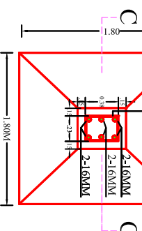
R.C.C. COL. FDN. PLAN SCALE 1:25
