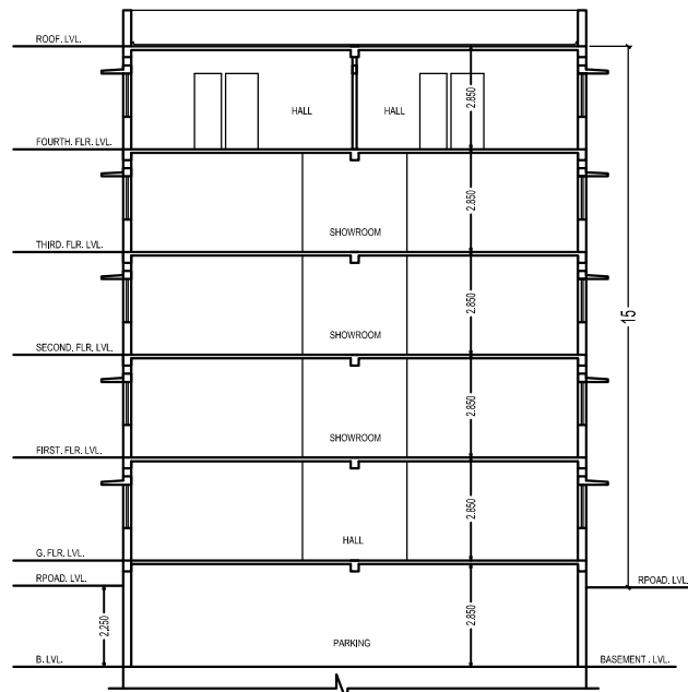
SECTION X-X SCALE: 1:100
