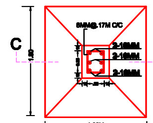
R.C.C. COL. FDN. PLAN SCALE 1:100
