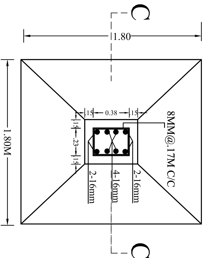
R.C.C. COL. FDN. PLAN SCALE - 1:25
