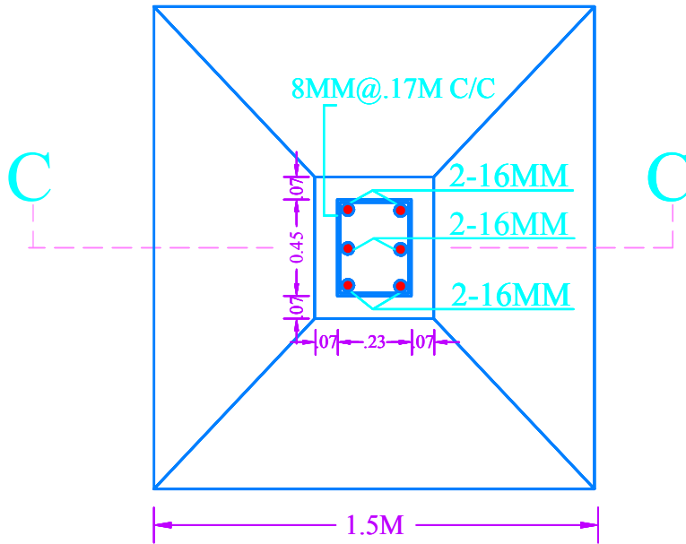
R.C.C. COL. FDN. PLAN
