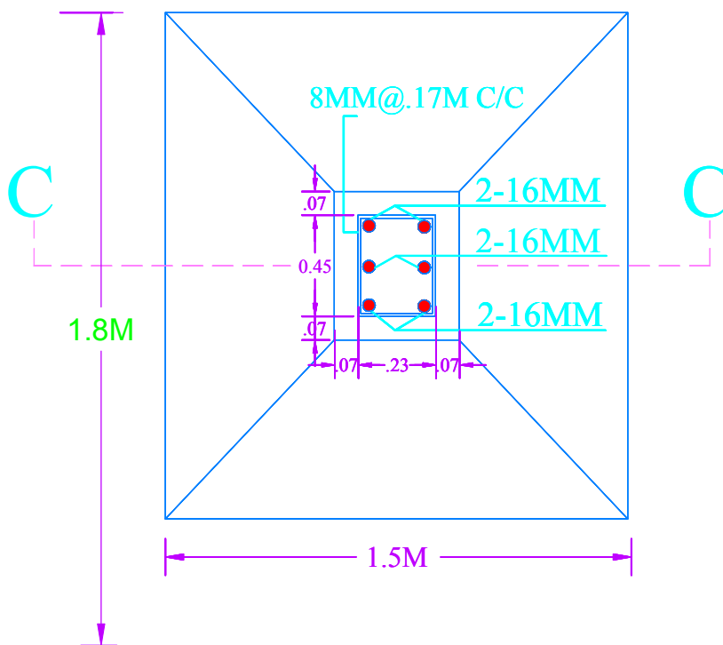
R.C.C. COL. FDN. PLAN
