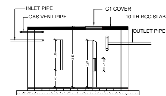
SECTION (N.T.S)
