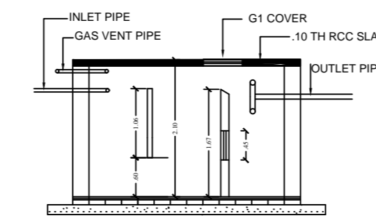
SECTION (N.T.S)
