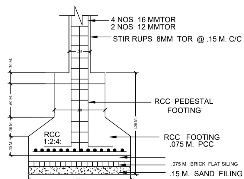
SECTION (N.T.S)
