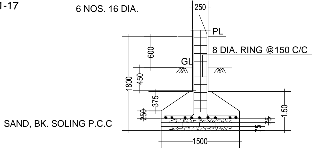
SECTION ON C-C SCALE - N.T.S
