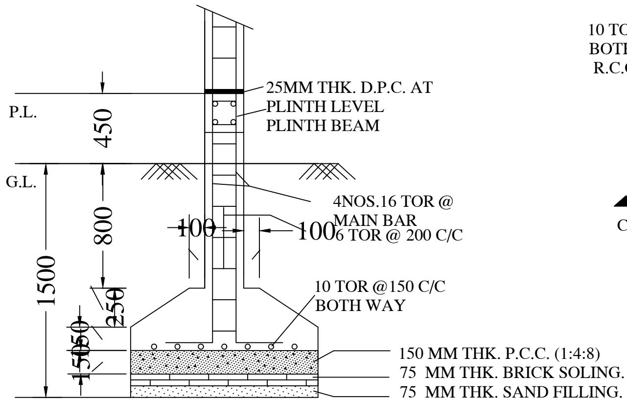
SECTION -CC
