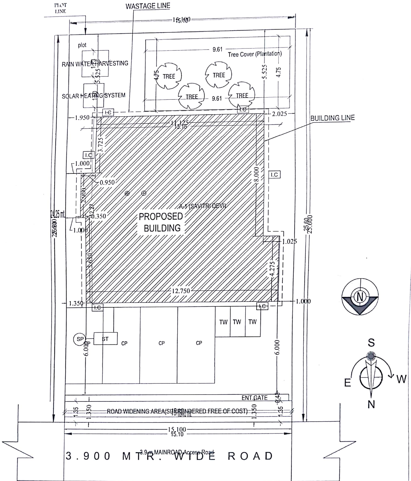
SITE PLAN PLAN SCALE 1:100
