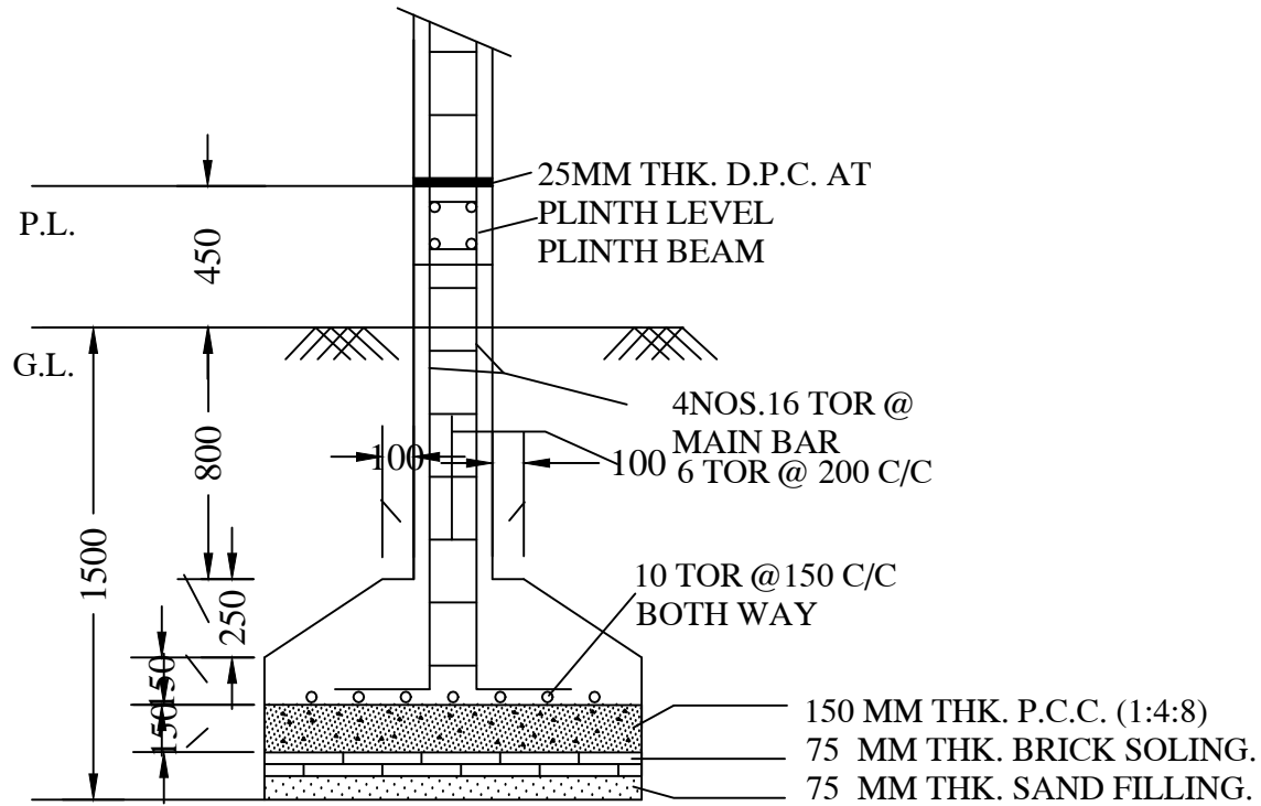
SECTION -CC
