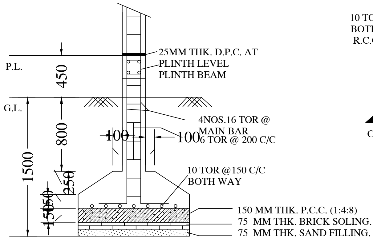
SECTION -CC
