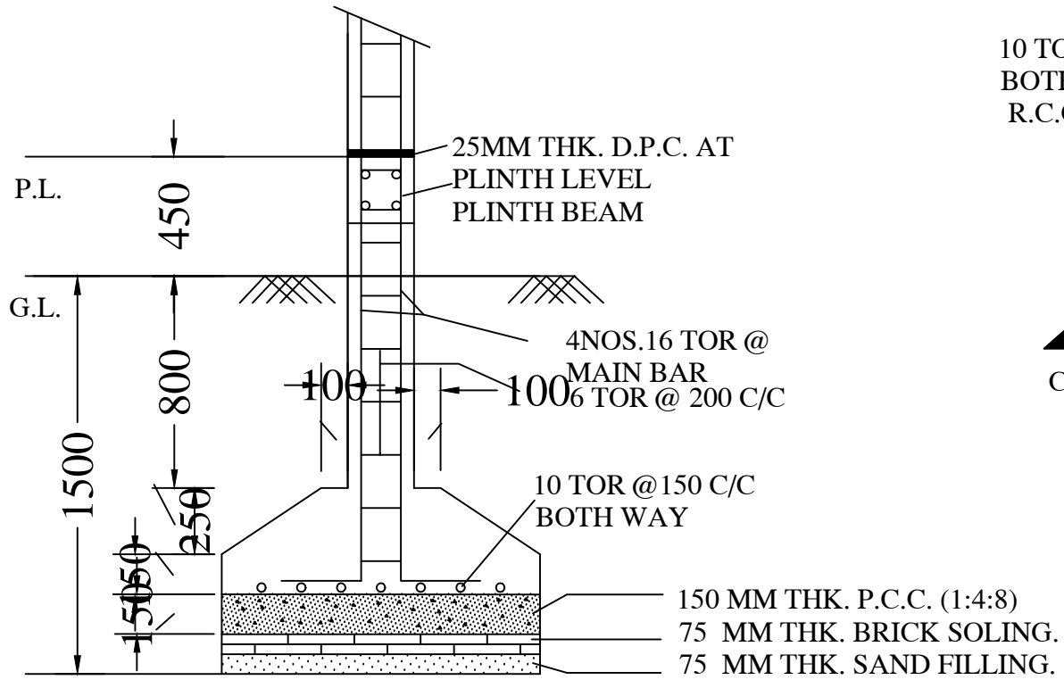
SECTION -CC
