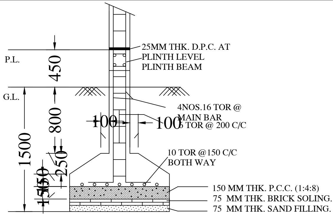
SECTION -CC
