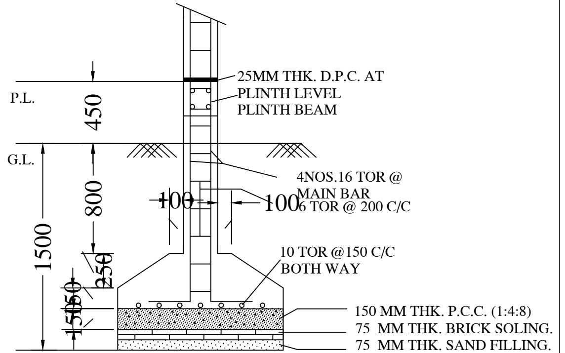
SECTION -CC
