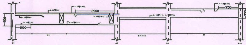
BEAM ALONG D1 - D7 - D8- D10 (300 X 500 & 250 X 350 )
