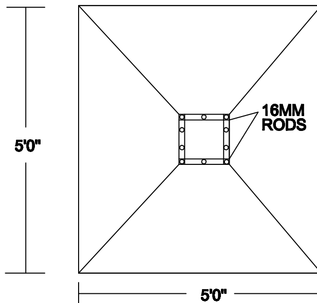
PLAN ( SCALE 1"=4')
