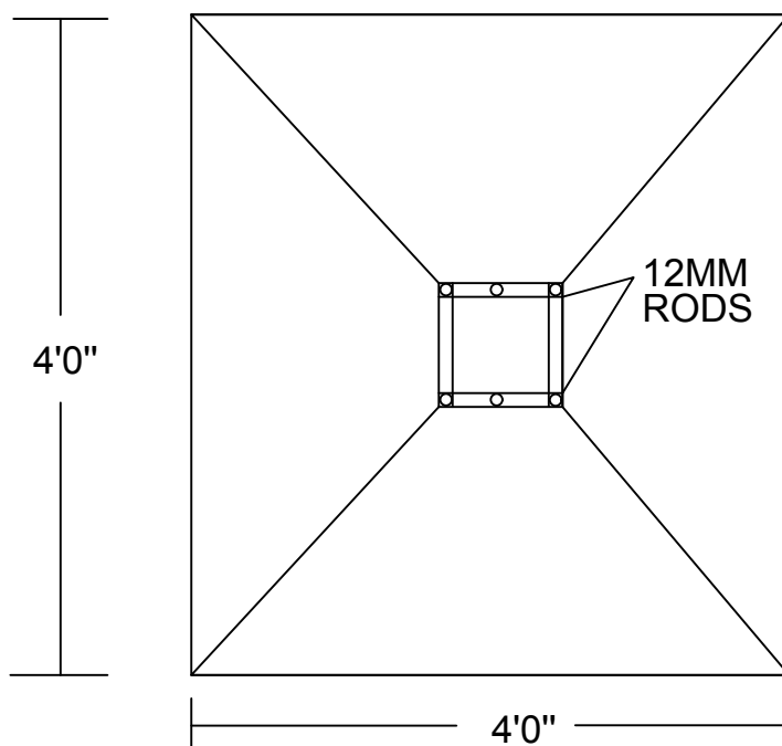
PLAN ( SCALE 1"=4')
