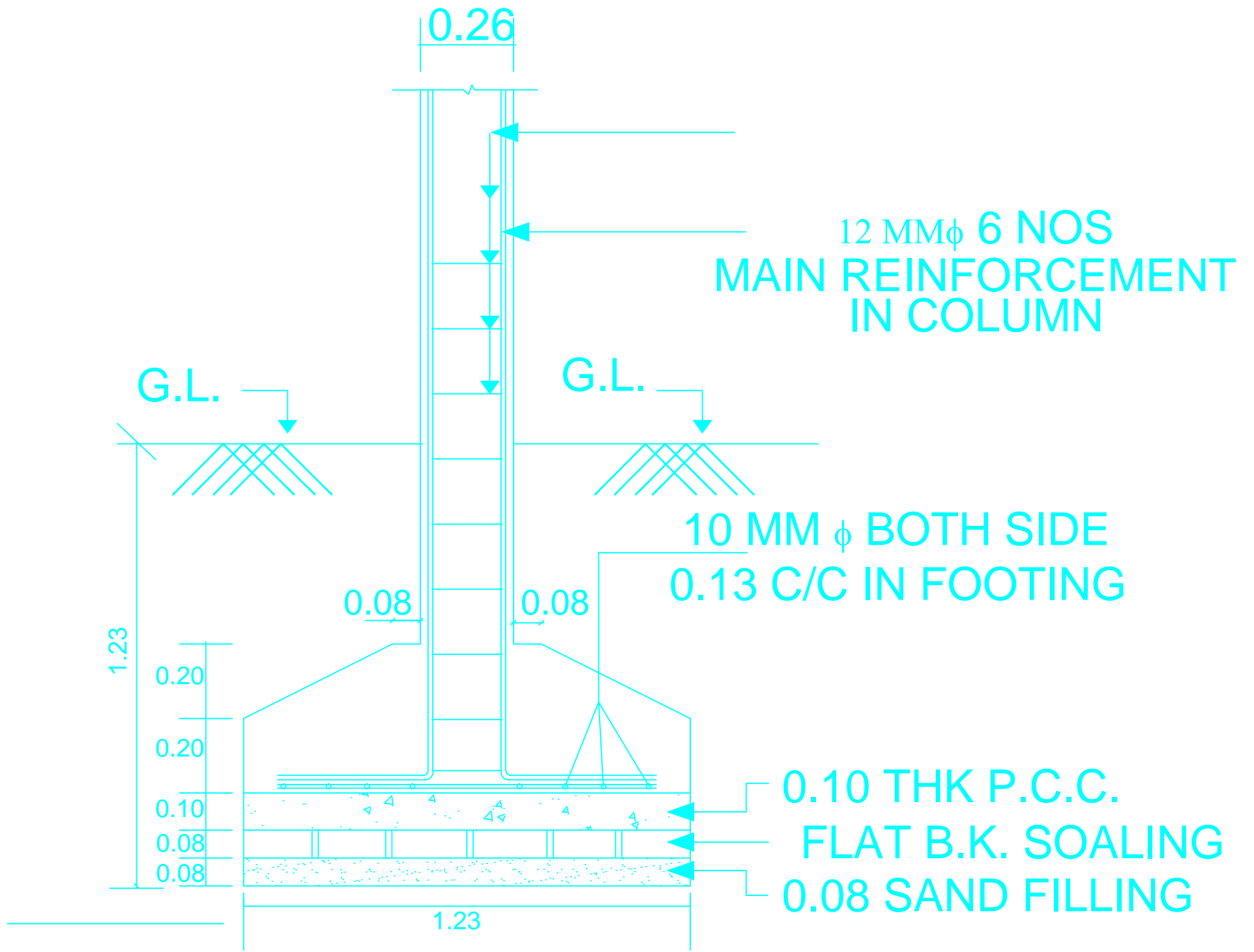
R.C.C. COLUMN
