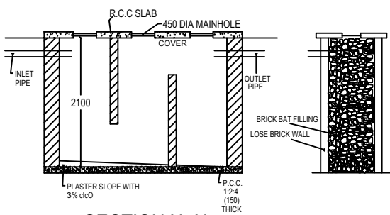
SECTION N.-N.
