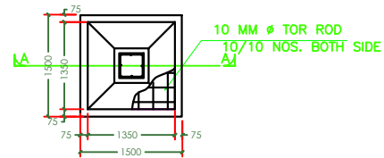
.COLUMN PLAN.
