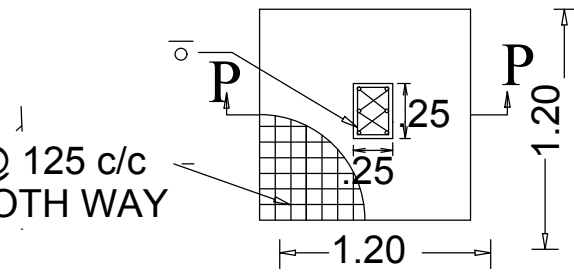
DET. OF COL. FDN.
