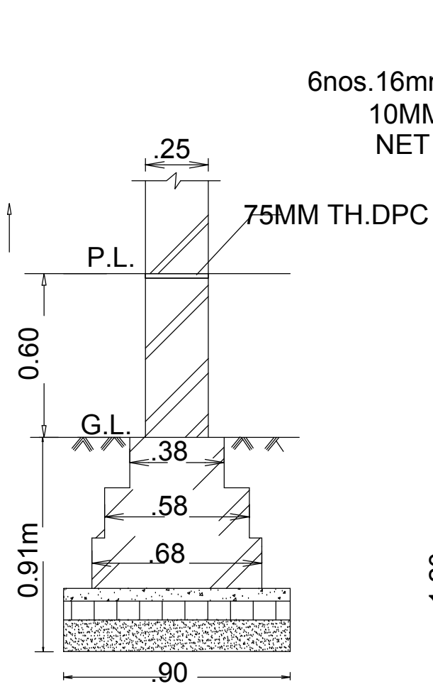
DET. OF FDN. SCALE -1:50
