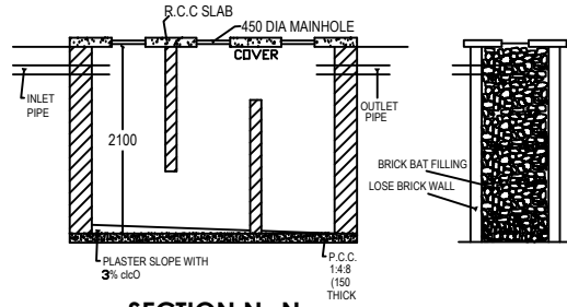
SECTION N-N.
