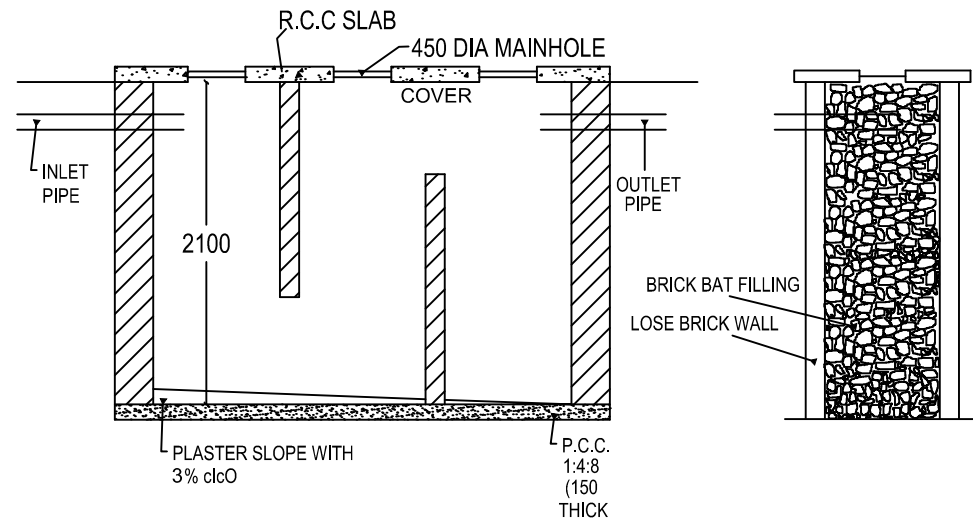
SECTION N.-N.
