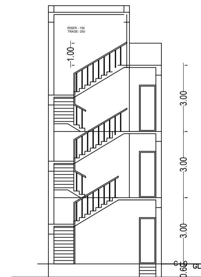
SECTION - A-A
