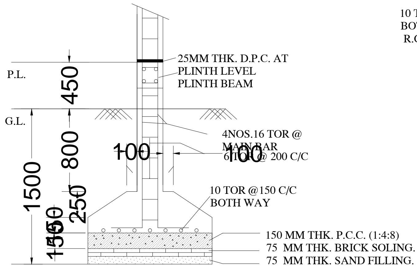
SECTION -CC
