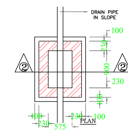
I.C.DETAILS
