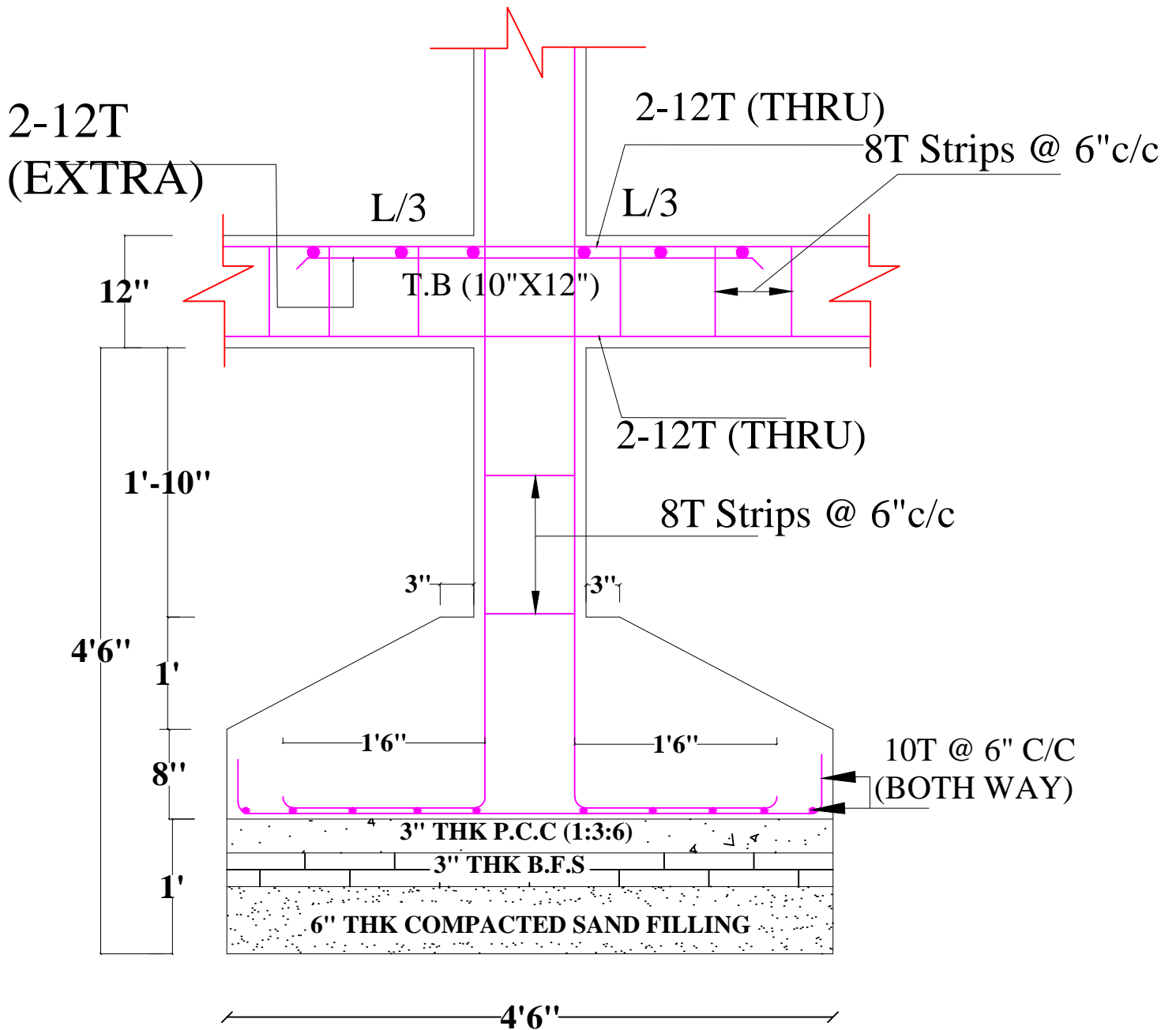
SECTION - D-D
