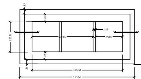
PLAN (N.T.S) DETAIL OF SEPTIC TANK
