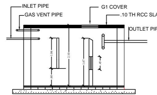
SECTION (N.T.S.)
