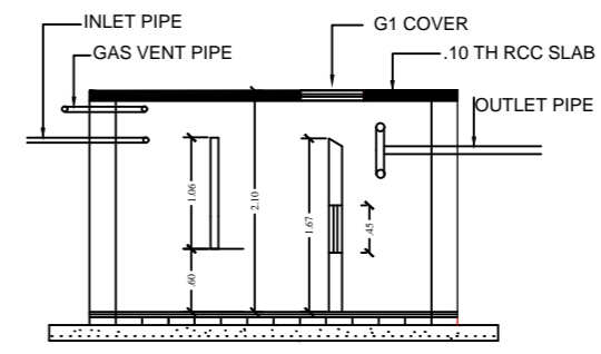
SECTION (N.T.S)
