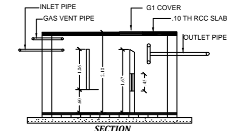
SECTION (N.T.S)
